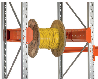
Jednotka pro výdej kabelů - se samosvornou osou. Nastavitelný uchycení bubnu a pohyblivá osa.
