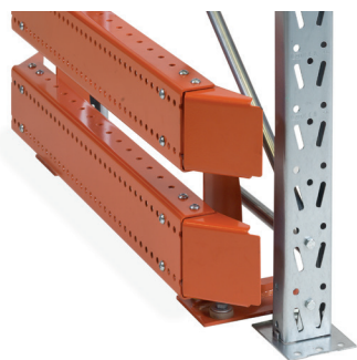
Ochrana rámu – pro koncový rám, stojiny a uličku pro vozíky. Pro jednotlivé i dvojité regály. Výška 400 mm.
