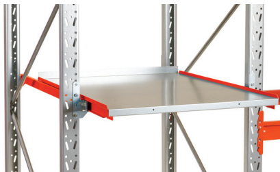
Výsuvná police pro pohodlné vychystávání nepaletizovaného zboží. Instalovaná na regálových stojinách.
